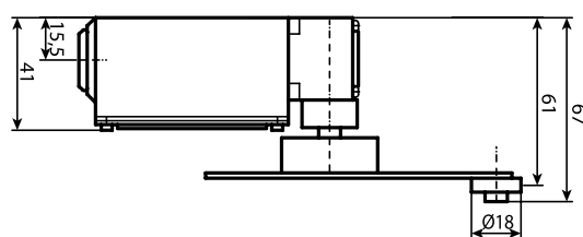
роликовый рычаг регулируемой длины
