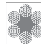
стальной трос 6х19
